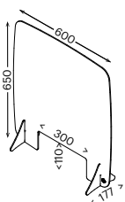
Pequeño modelo sobre pies
