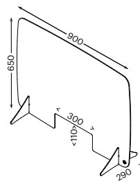
Grande modelo sobre pies
